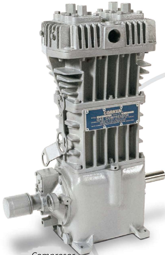
Compresor Modelo 491
